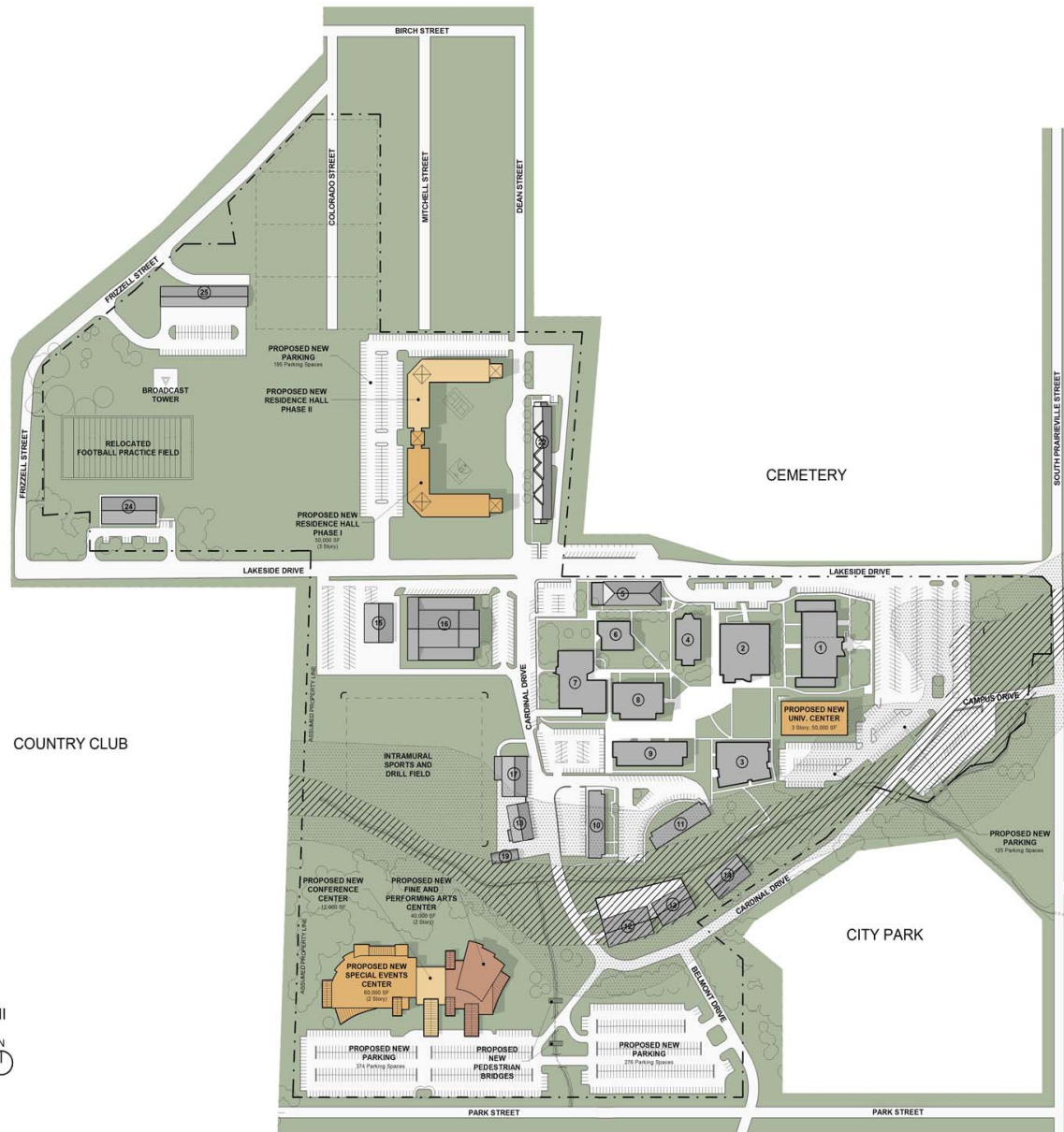
SITE PLAN--PHASE III
